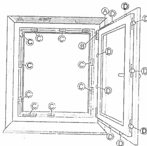
obr. 1: Přehled pozic pro mazání
