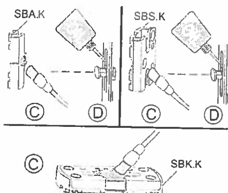
obr. 3: Protiplechy
