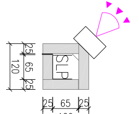
DETAIL 04 - STOJKA NA POHYBOVÉ ČIDLO
