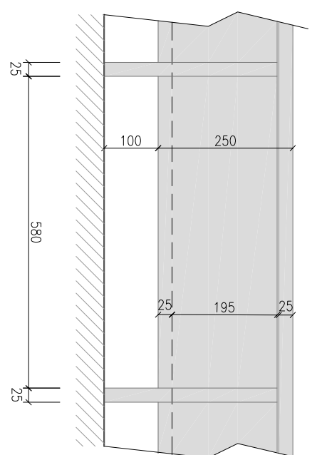
DETAIL 02 - ENERGOKANÁLEK SCHODIŠŤOVÝ 150x250 mm
