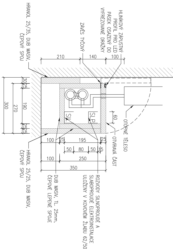
ŘEZ
