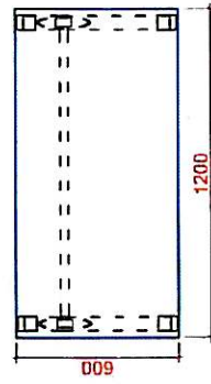
S6-12 podlož. kovová samonosná středová 35 mm podlož. RAL 9006
