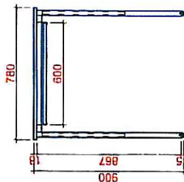
SPC hl. 600 mm podnož je 30/30 RAL 9006 zástěpy s rektifikací DTD-L VÝPLNĚ VKD 5.500 mm
