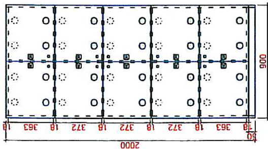
AT BOT hloubka 398 mm 10x zámek (každý jiný) 10x knopka 20x vrtáček 20x otvor v zádech
