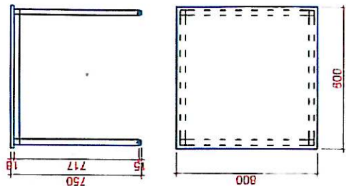
SU-80 podnož je 30/30 zástěpy s rektifikací RAL 9006
