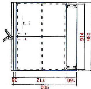
KL 95 hloubka 500 mm PD TL 38 mm krycí listy dřez s odkapem boletin
