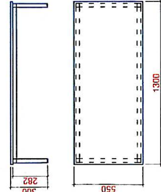
POD JEKL 30/30 RAL 9005
