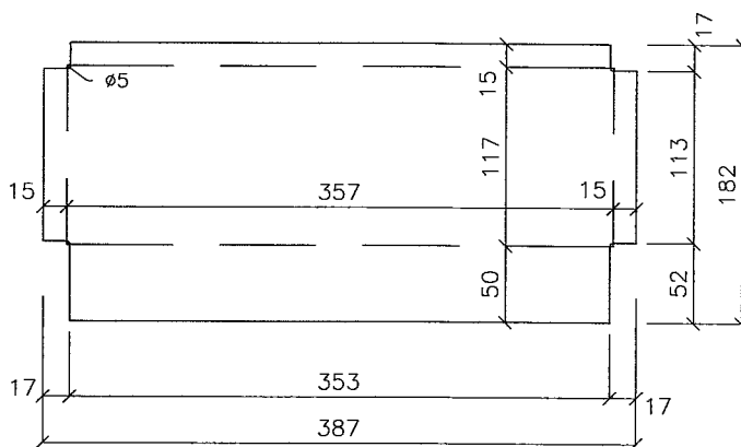
8.257 DNO – ROZVINUTÝ TVAR
