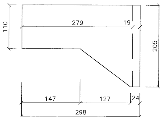
8.256 BOK – ROZVINUTÝ TVAR
