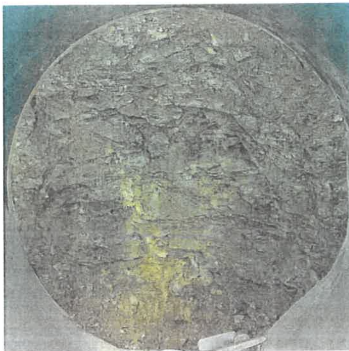
Obrázek V. – čelba m 7,2
